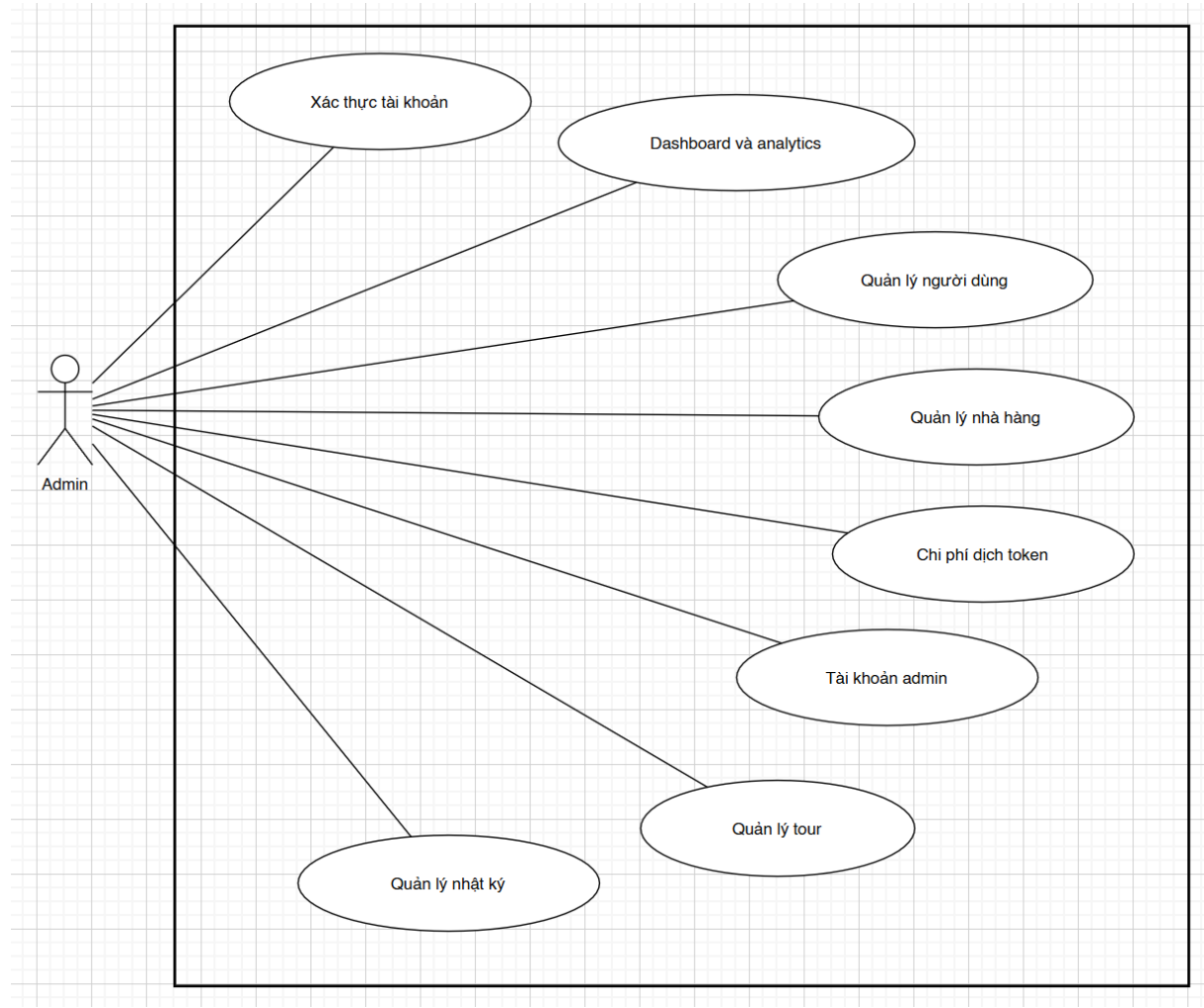
TongQuat.png
