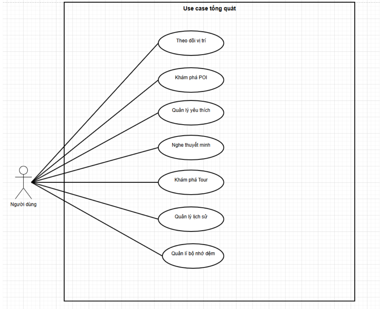
TongQuat.png
