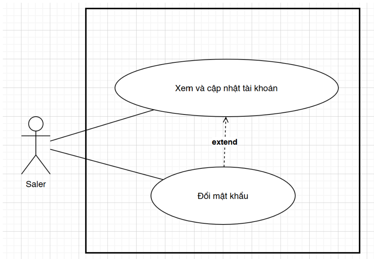
TaiKhoan.png
