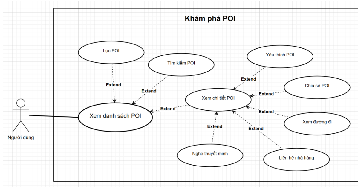
KhamPhaPOI.png
