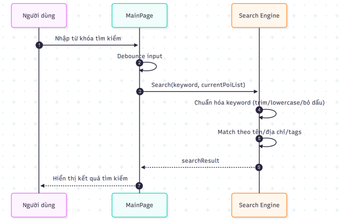
TimKiemPOi.png
