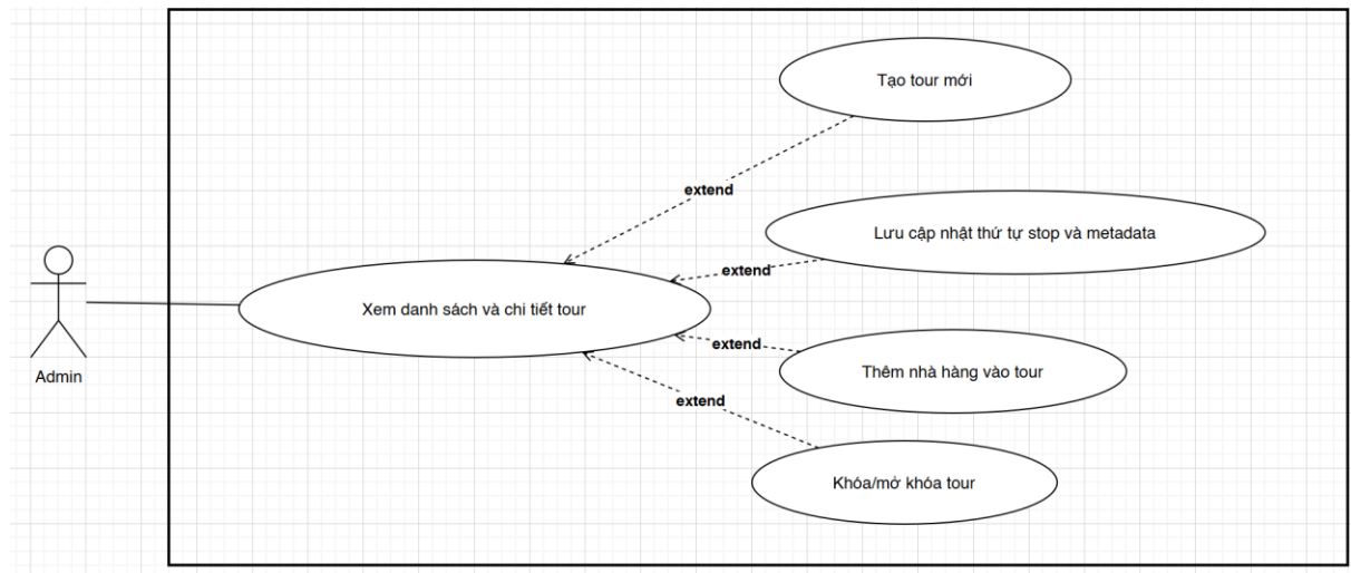
Tour.png
