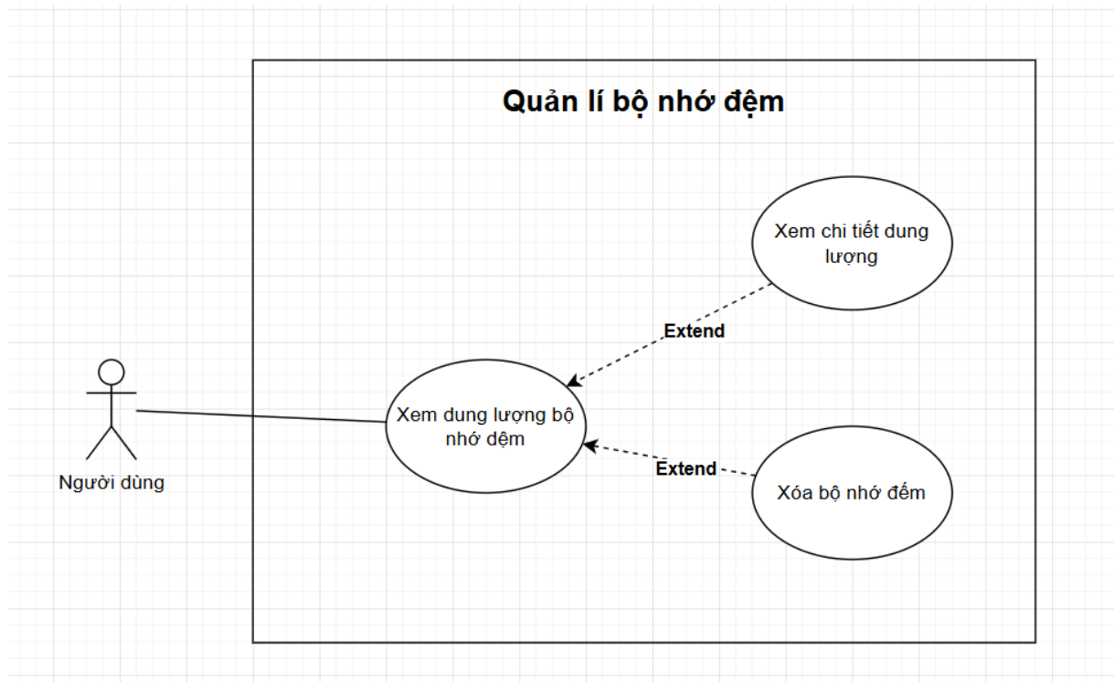
QuanLiBoNhoDem.png
