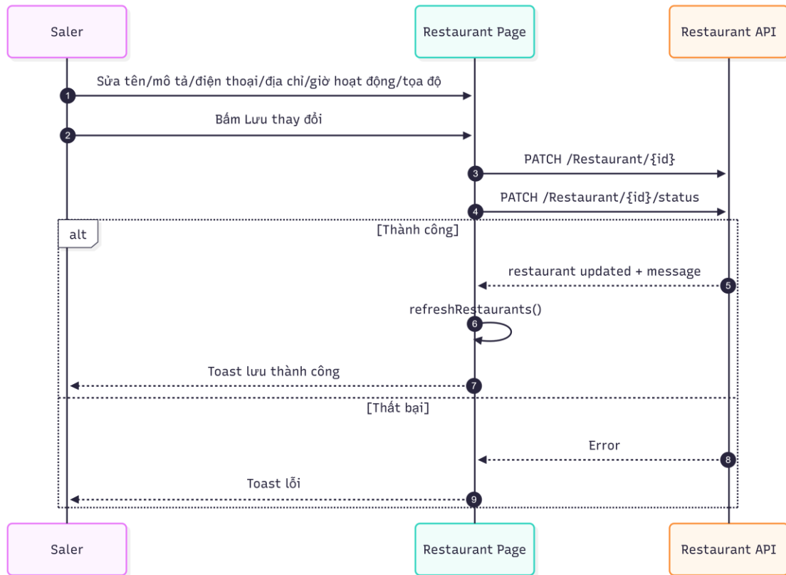
8_CapNhatThongTinNhaHang.png
