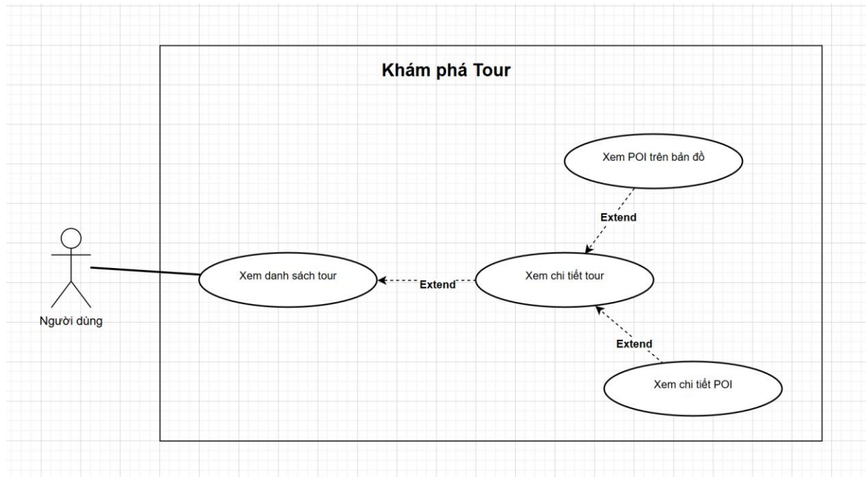
KhamPhaTour.png
