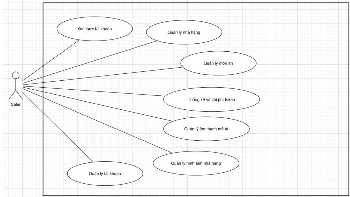
TongQuat.png
