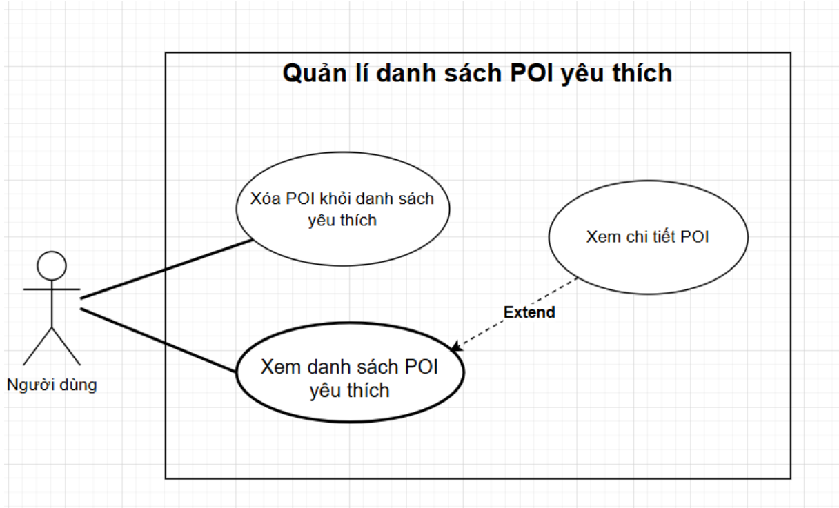
QuanLiDanhSachYeuThich.png
