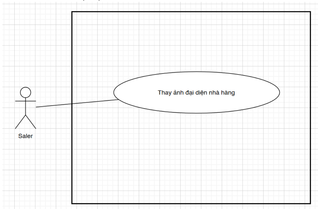
AnhDaiDien.png
