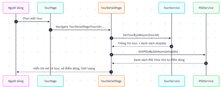
XemChiTietTOUR.png
