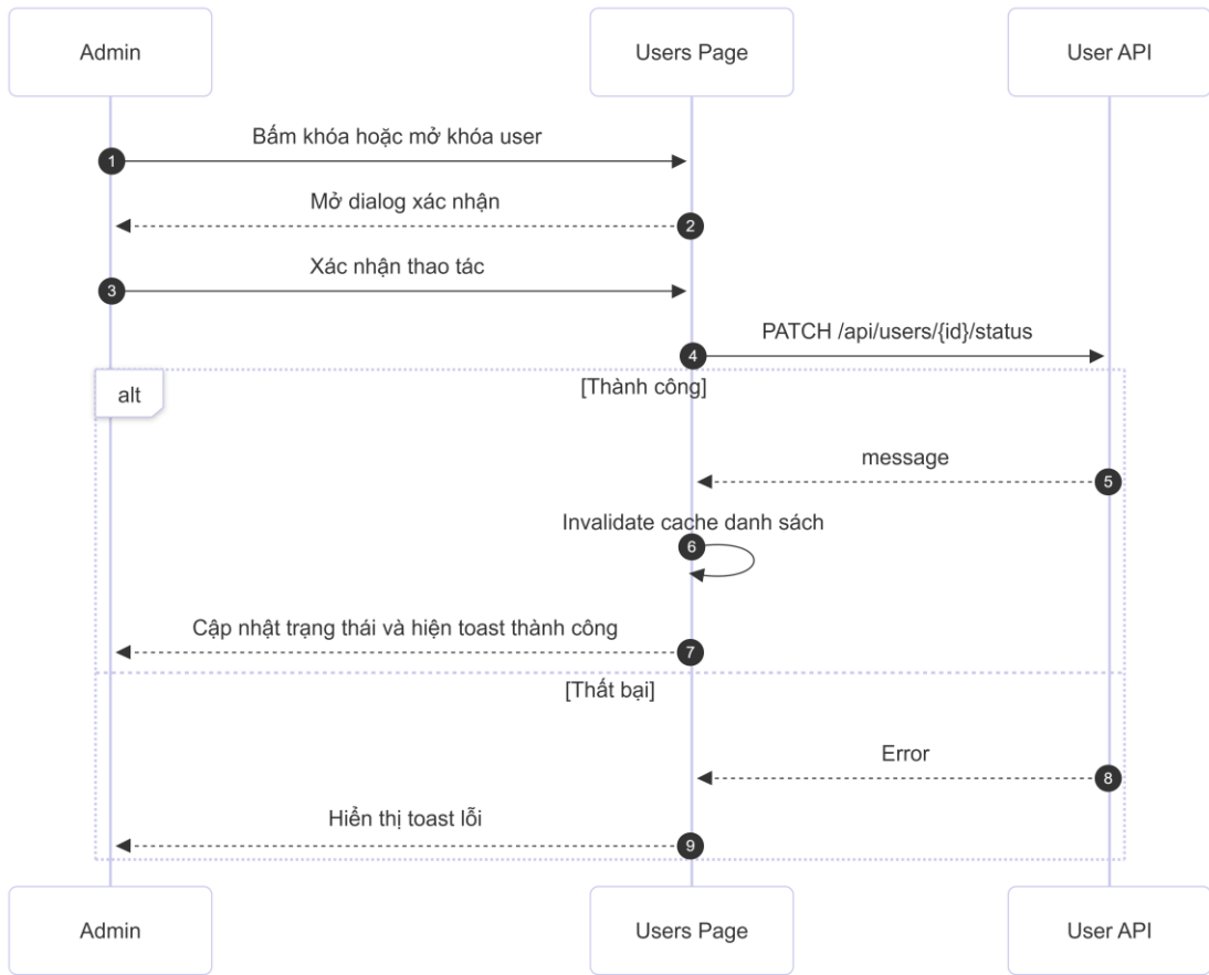
14_KhoaNguoiDung.png
