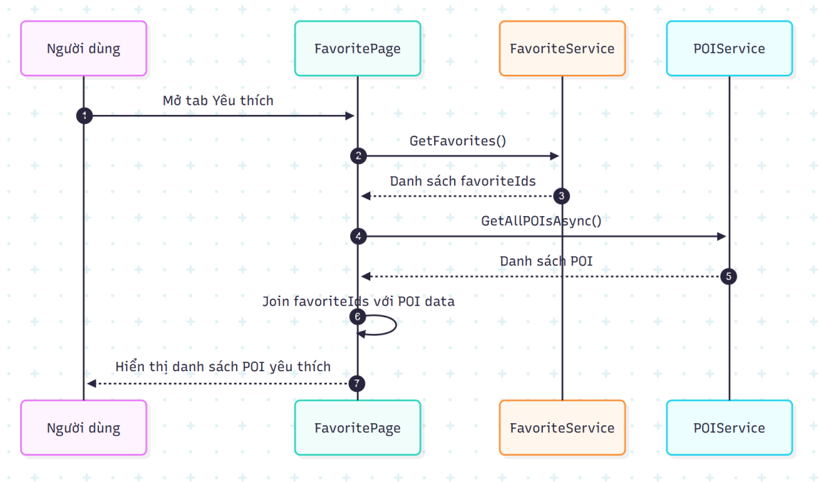
XemDSPOIYeuThich.png
