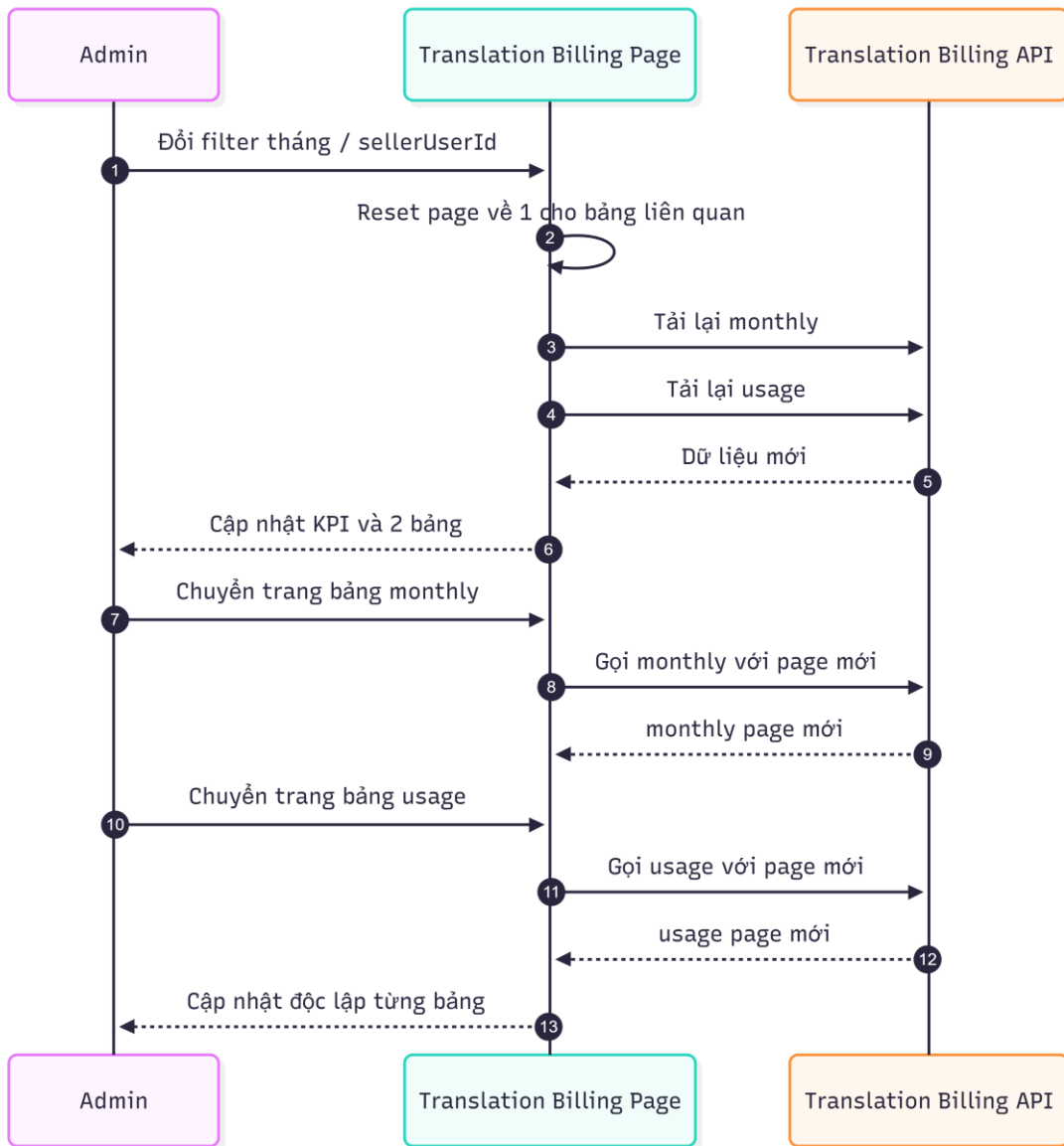
24_LocVaPhanTrangDich.png
