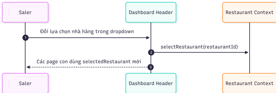
6_ChonNhaHangDeQL.png
