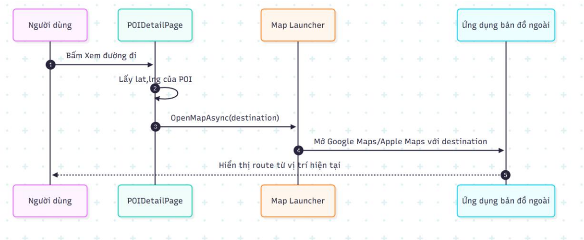
XemDuongDi.png
