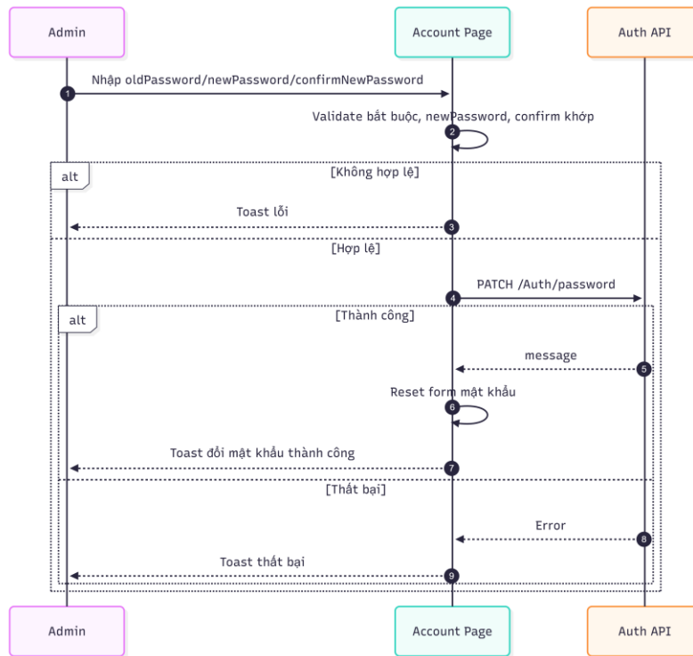
22_DoiMatKhauMoTaiKhoan.png
