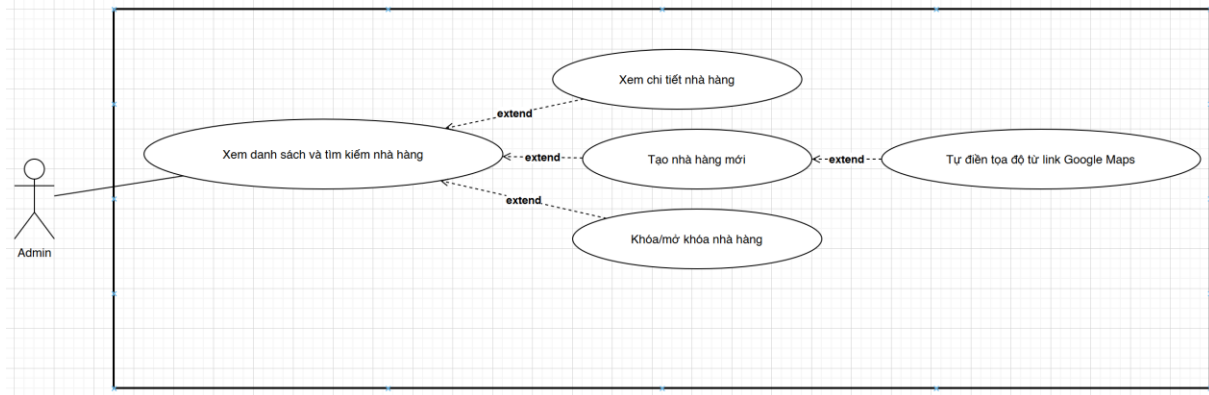
DanhSachNhaHang&TimKiem.png
