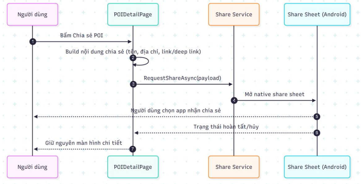
ChiaSePOI.png
