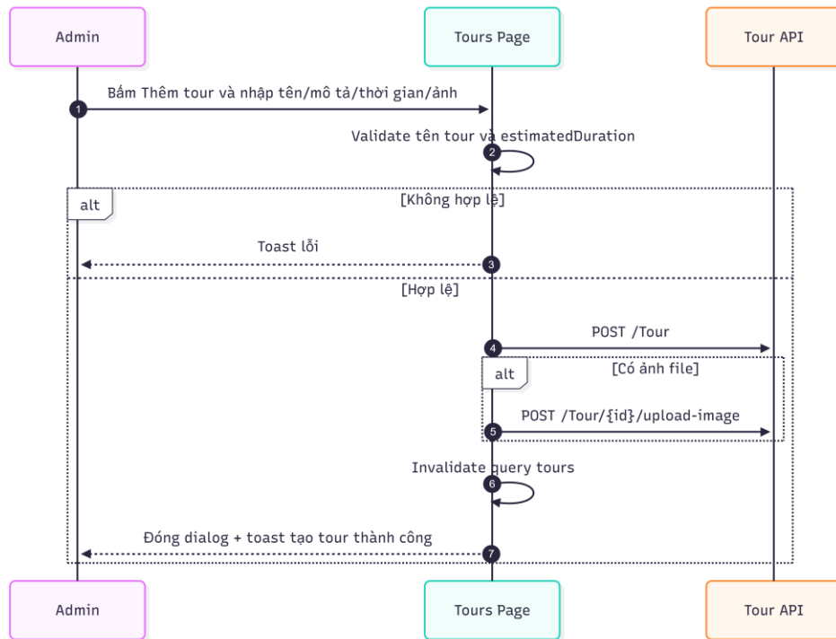
18a_TaoTourMoi.png
