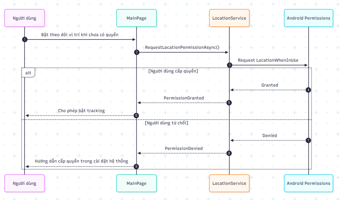
XinQuyentruyCap.png
