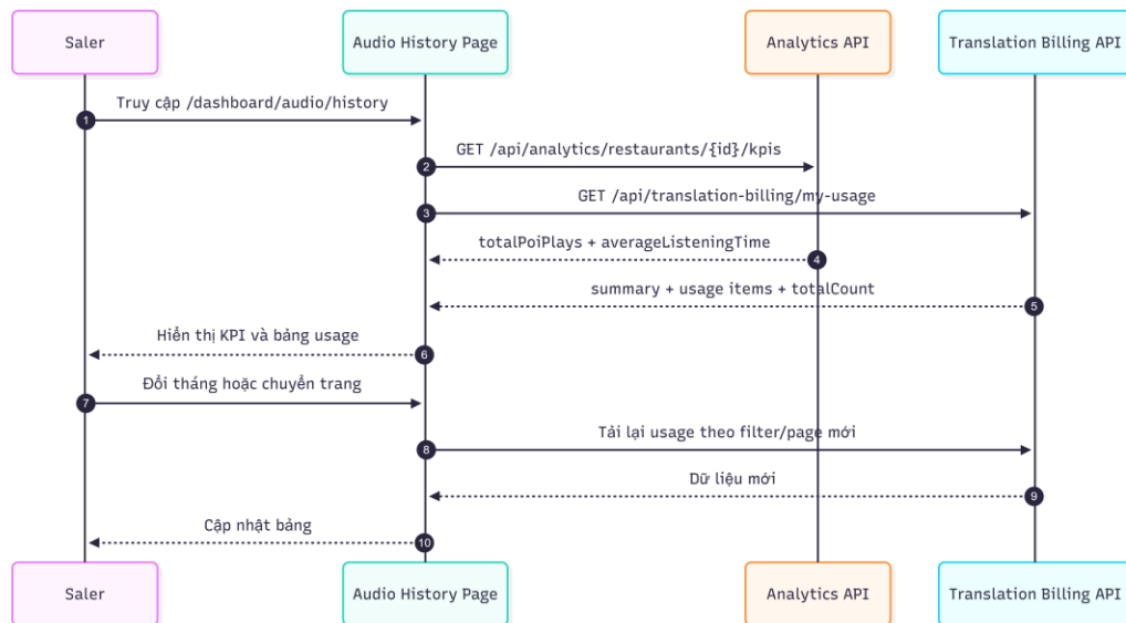
18_XemThongKeVaLichSu.png
