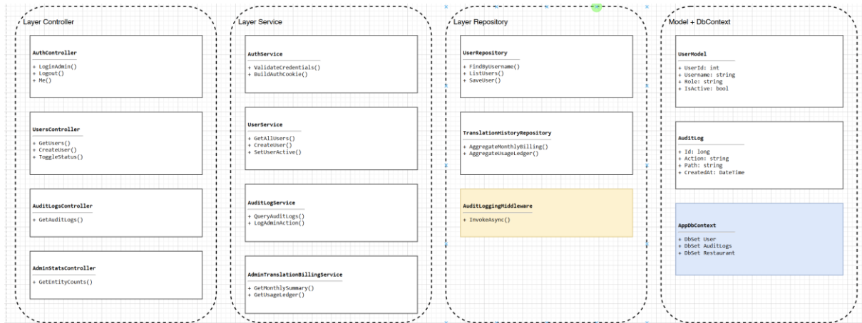
class_admin.png
