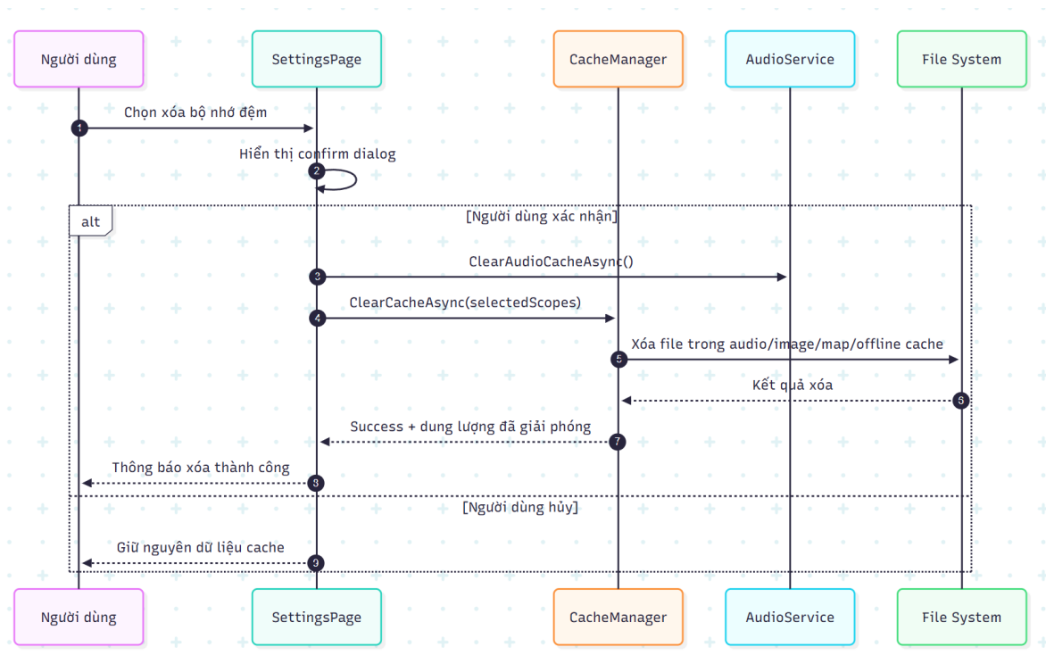
XoaBoNhoDem.png
