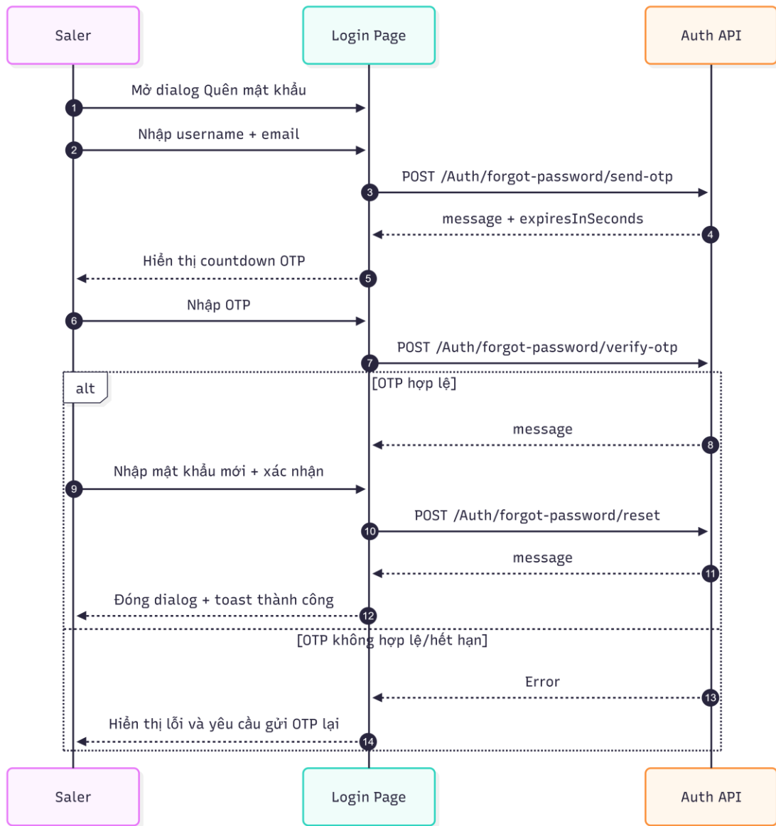
3_QuenMatKhau.png
