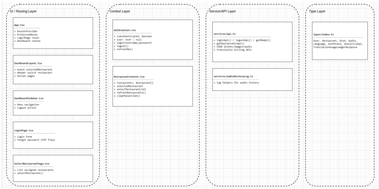
Class_saler.png
