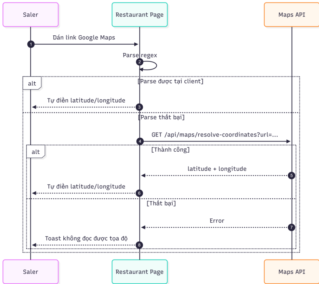
10_TuDienToaDo.png
