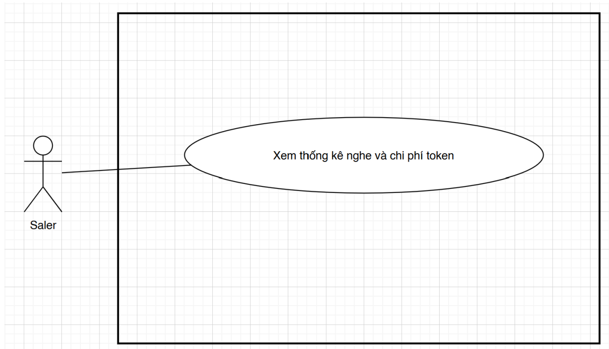
ThongKe.png
