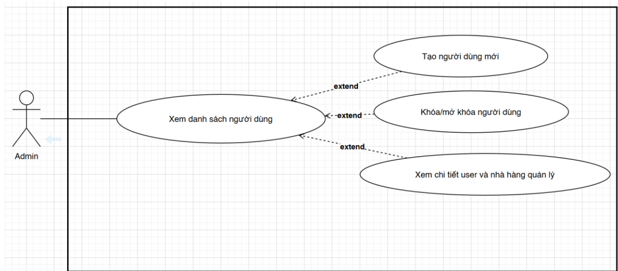
NguoiDung.png
