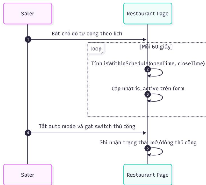
8_CapNhatThongTinNhaHang.png
