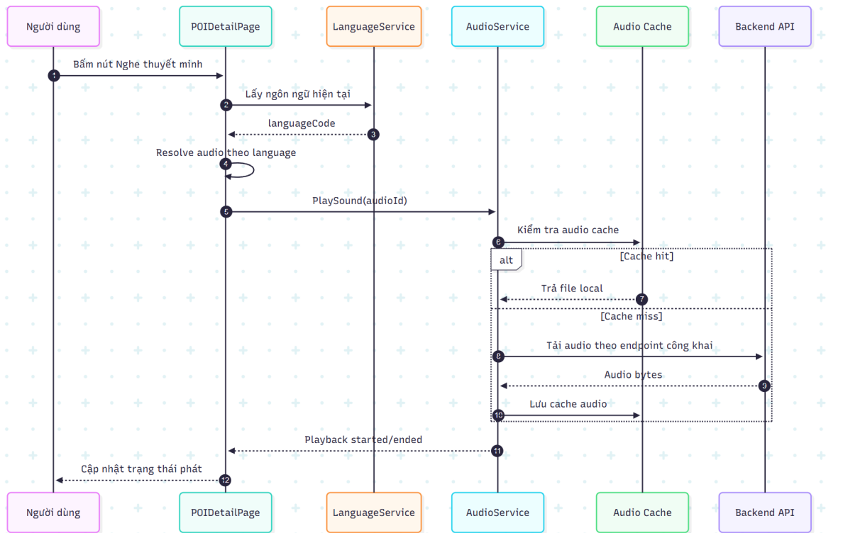
NgheThuyetMinh.png
