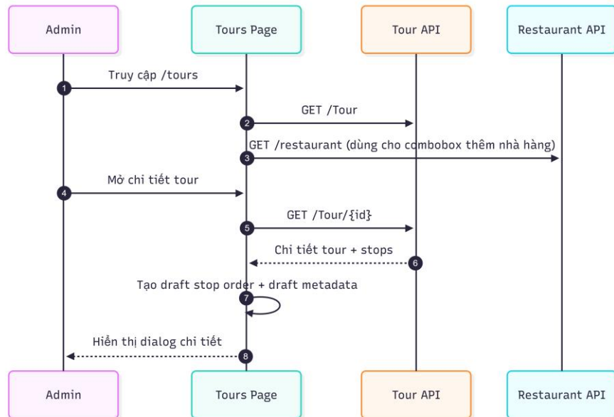
18_XemChiTietTour.png
