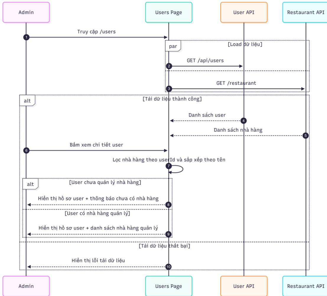
14a_XemChiTietNhaHang&NguoiDungQuanLy.png
