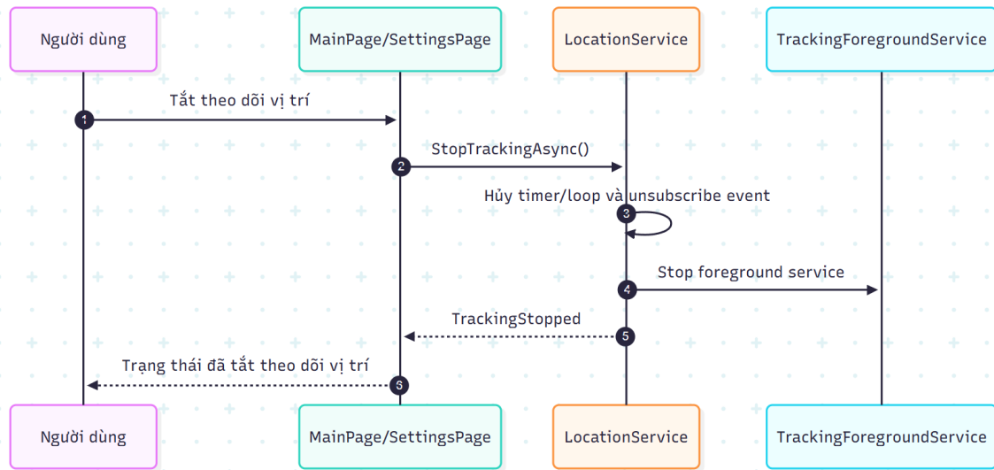
TatTheoDoiViTri.png
