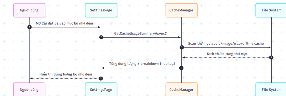
XemDungLuongBoNhoDem.png
