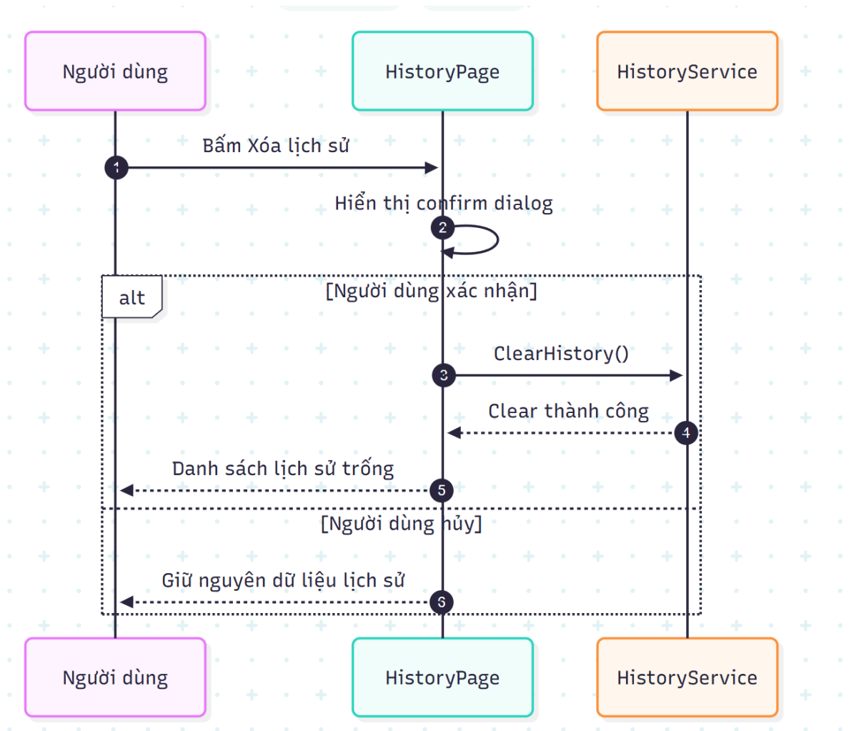
XoaLichSu.png
