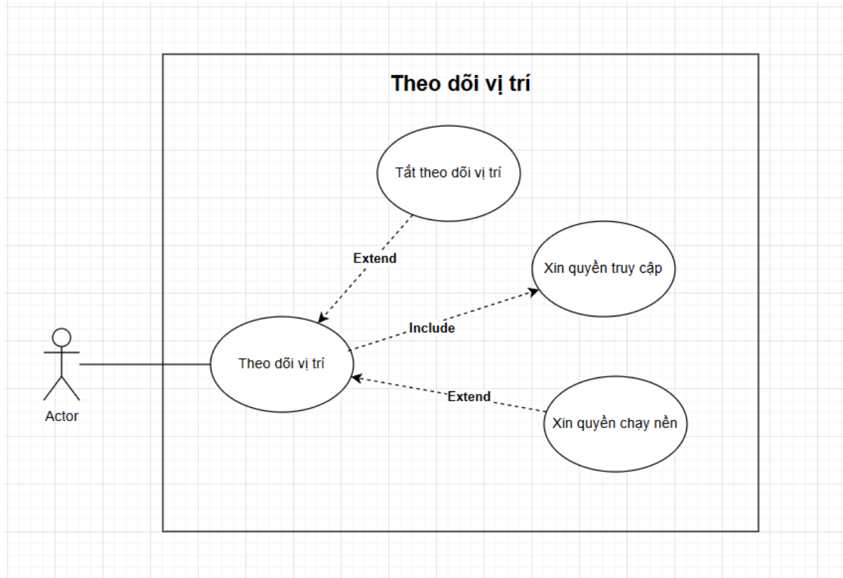
TheoDoiViTri.png
