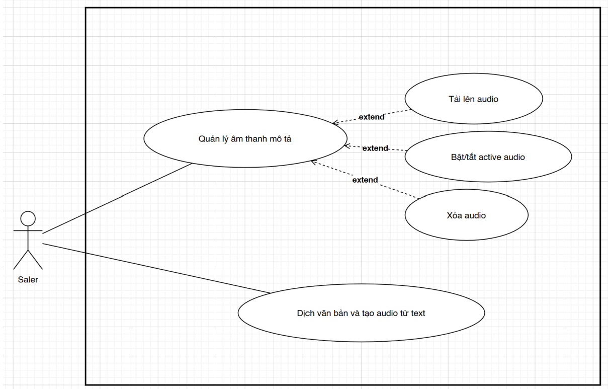
AmThanh.png
