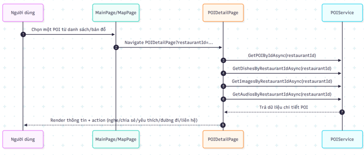
XemChiTietPOI.png
