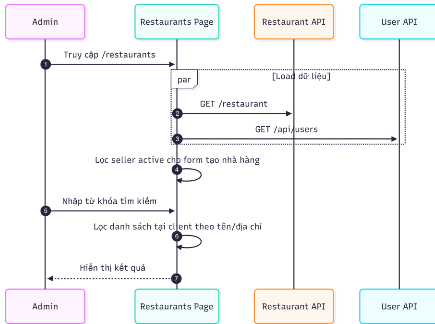
8_TimKiemVaHienNhaHang.png
