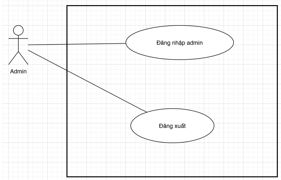
DangNhap.png
