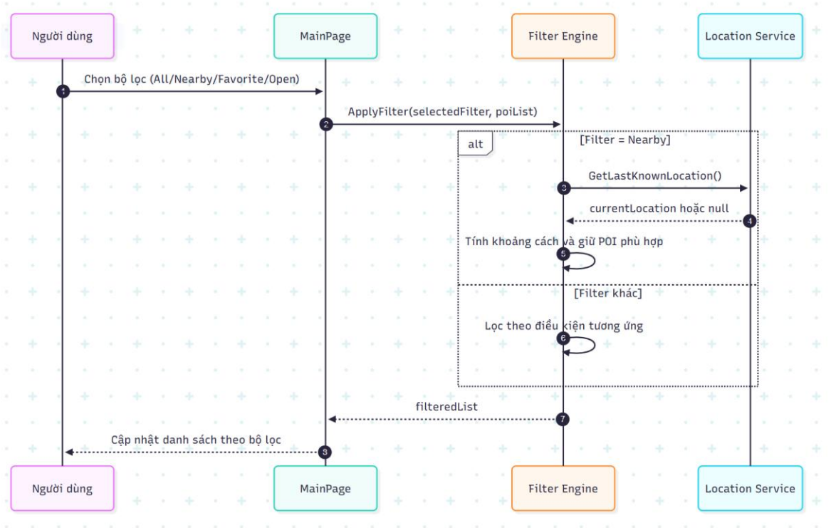
LocPOI.png
