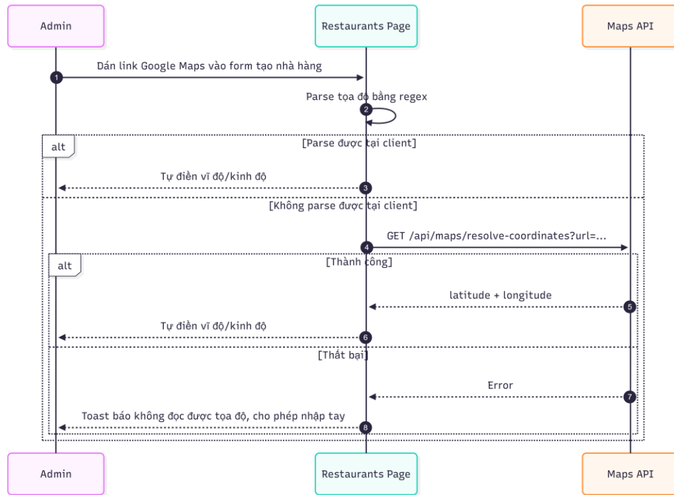
10a_DienToaDoaGMap.png
