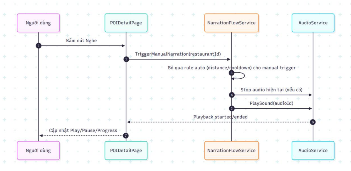
NgheThuyetMinhThuCong.png
