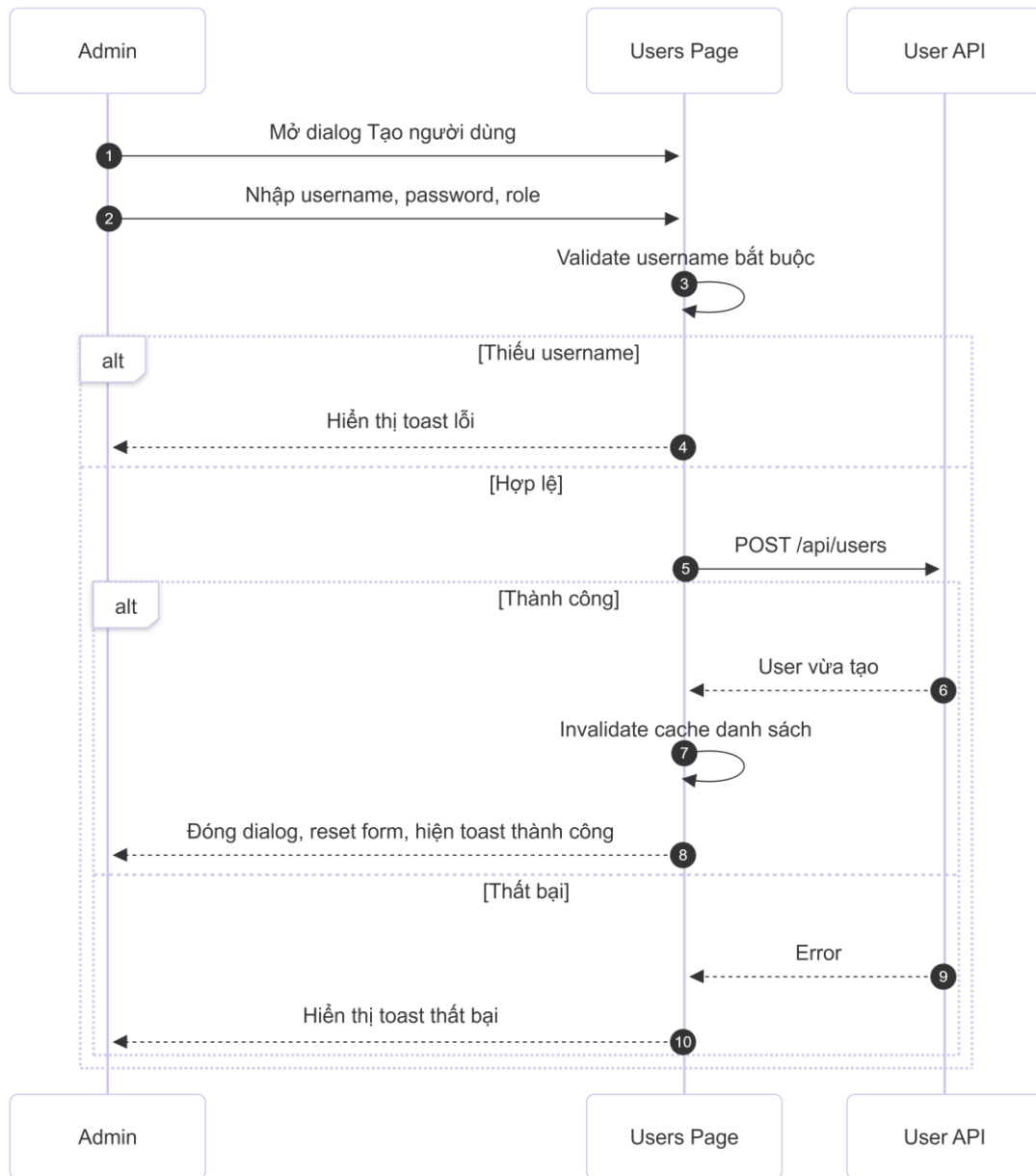
13_ThemNguoiDung.png
