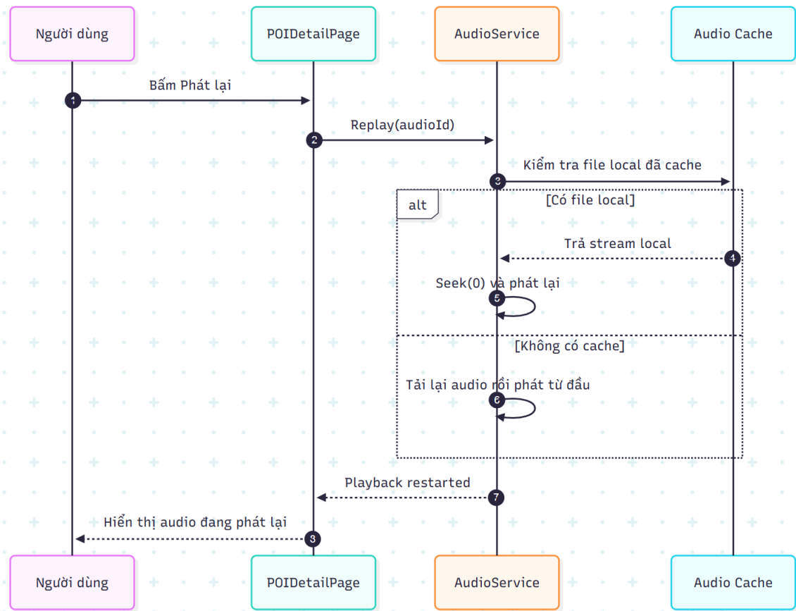
PhatLaiAudio.png
