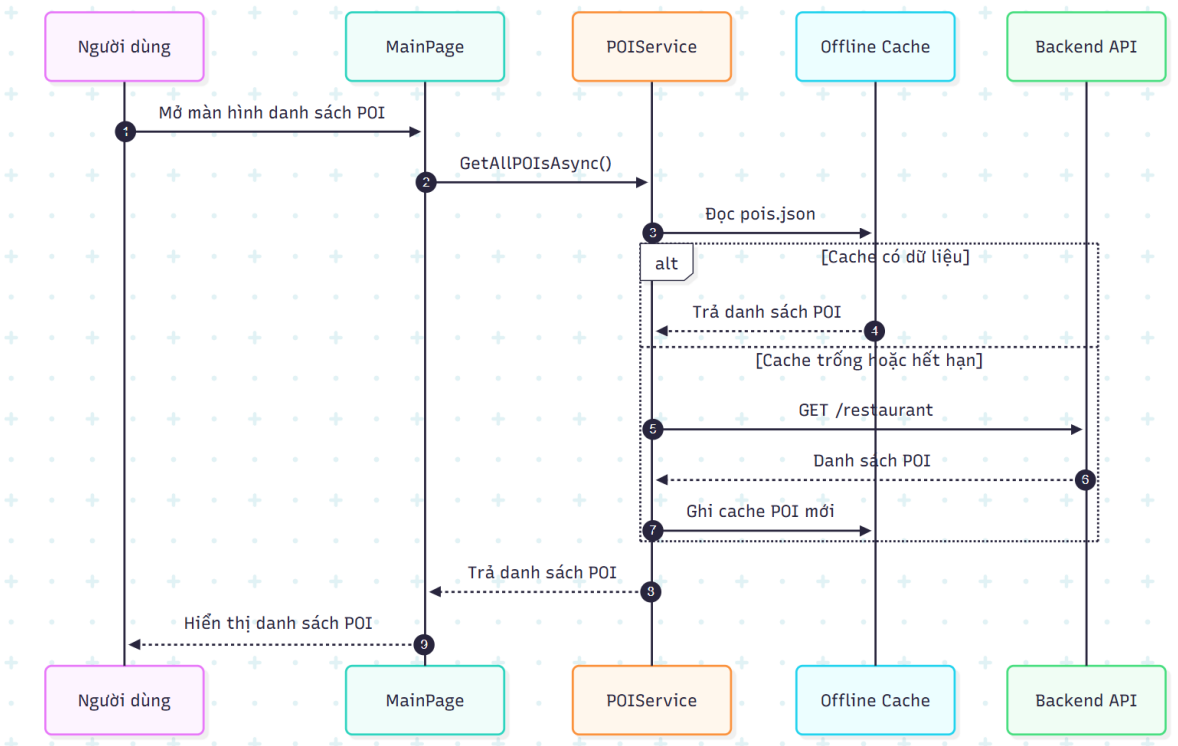
XemDanhSachPOI.png
