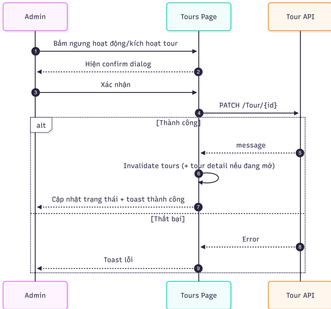
20a_KhoaTour.png
