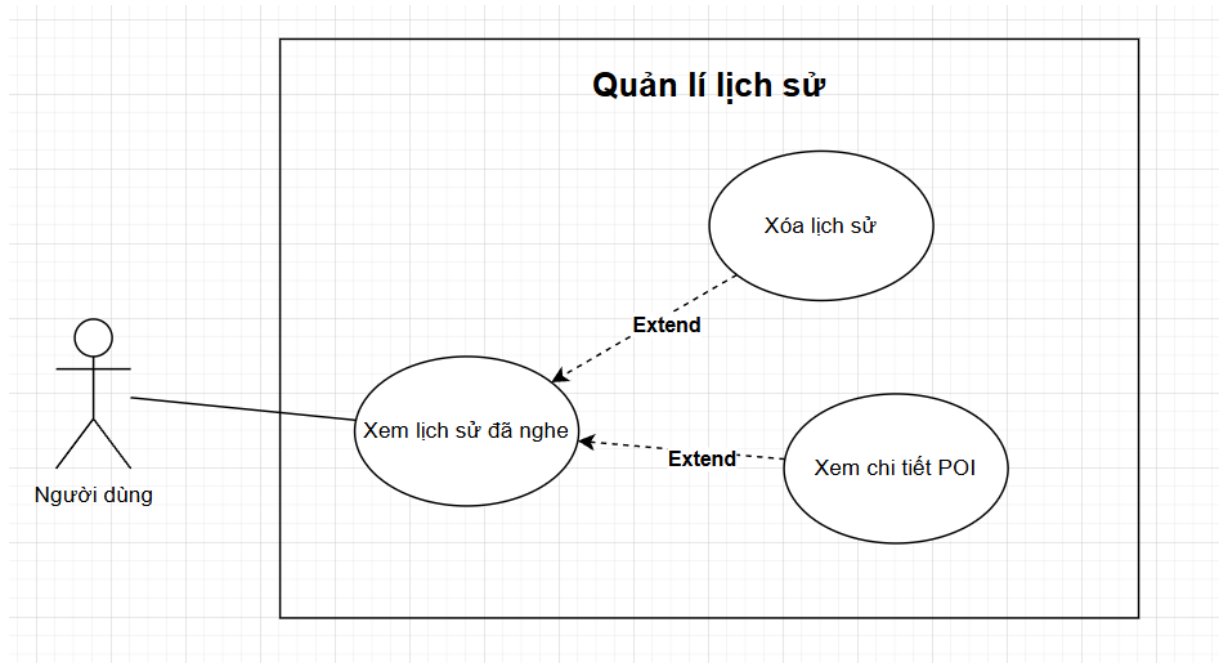
QuanLiLichSu.png
