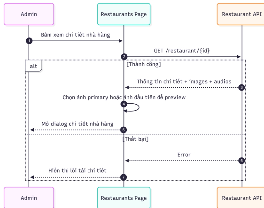
8_TimKiemVaHienNhaHang.png
