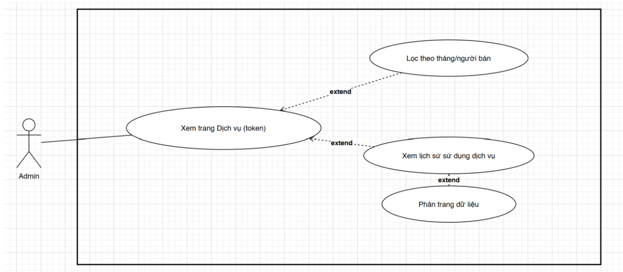
QuanLyDich.png
