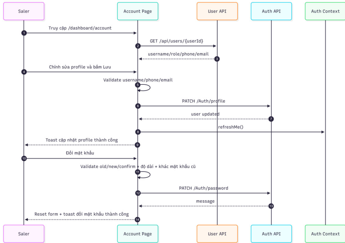
19_XemVaCapNhatTaiKhoan.png
