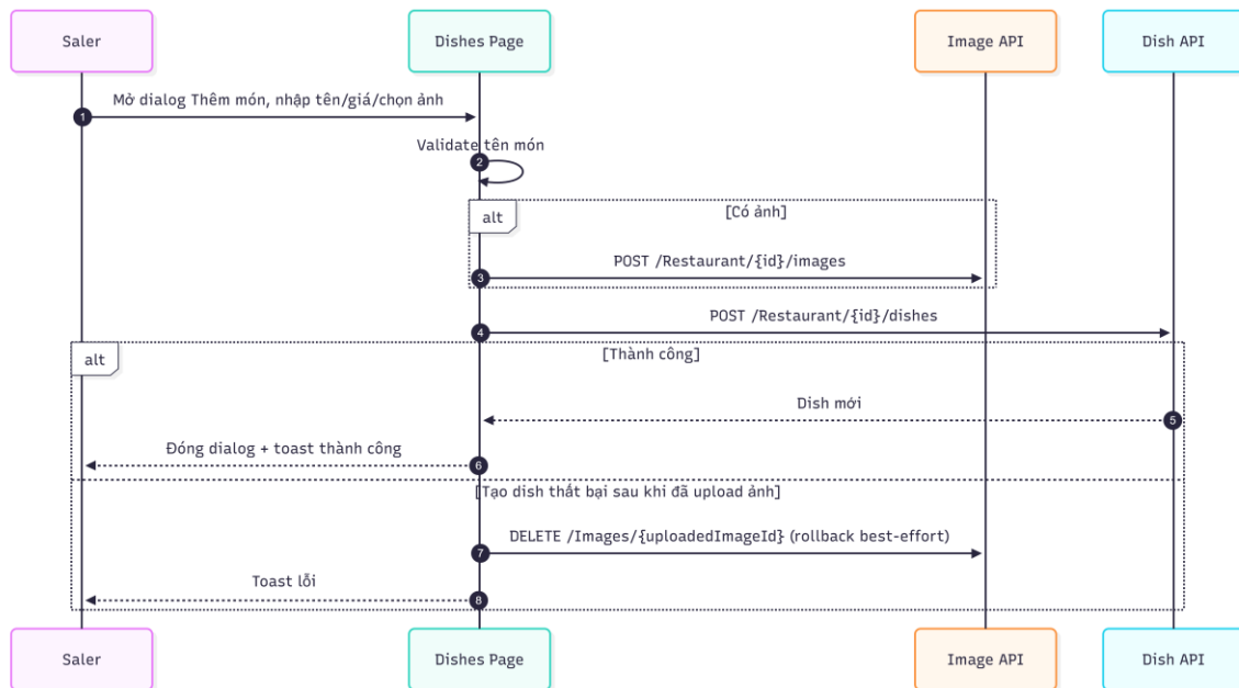
12_ThemMonAnMoi.png
