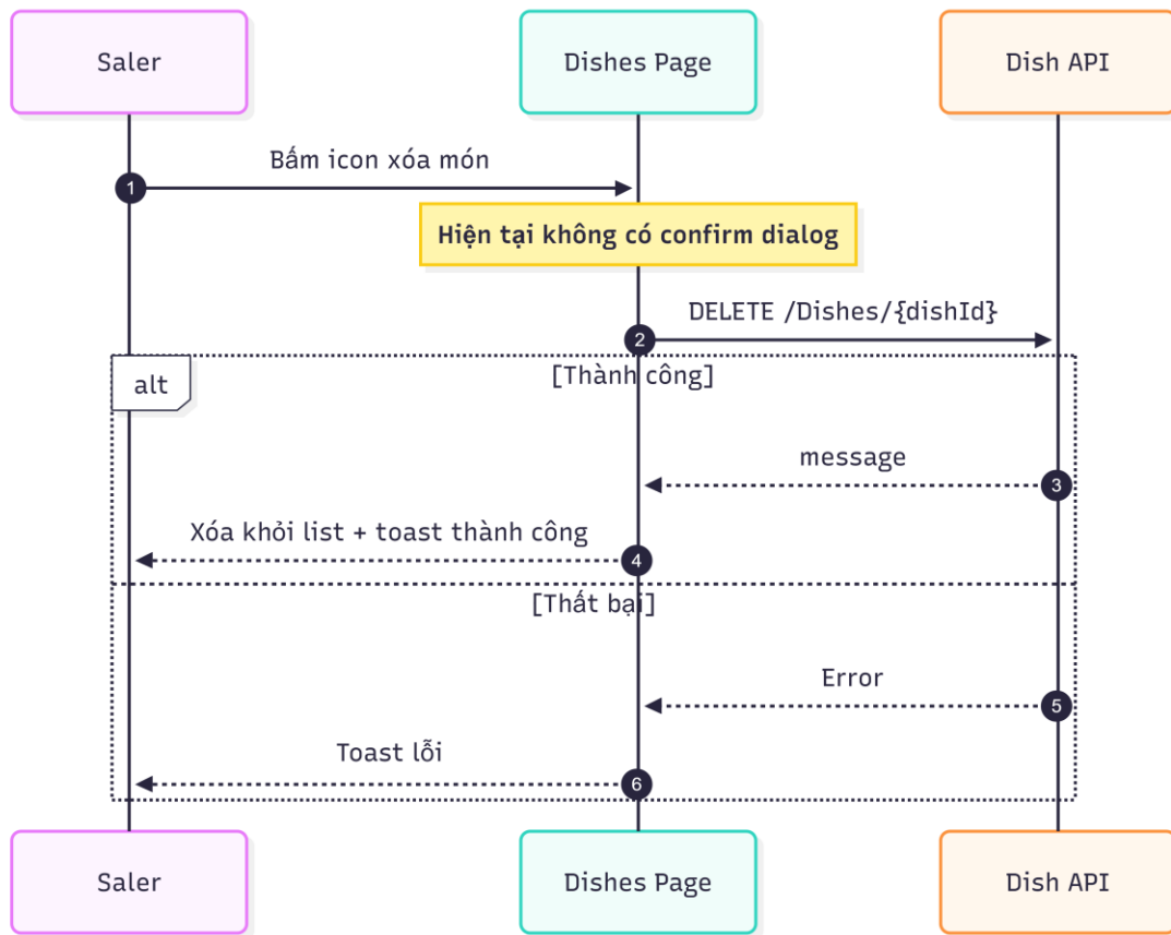
14_XoaMonAn.png
