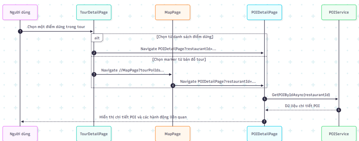
XemChiTietPOI.png
