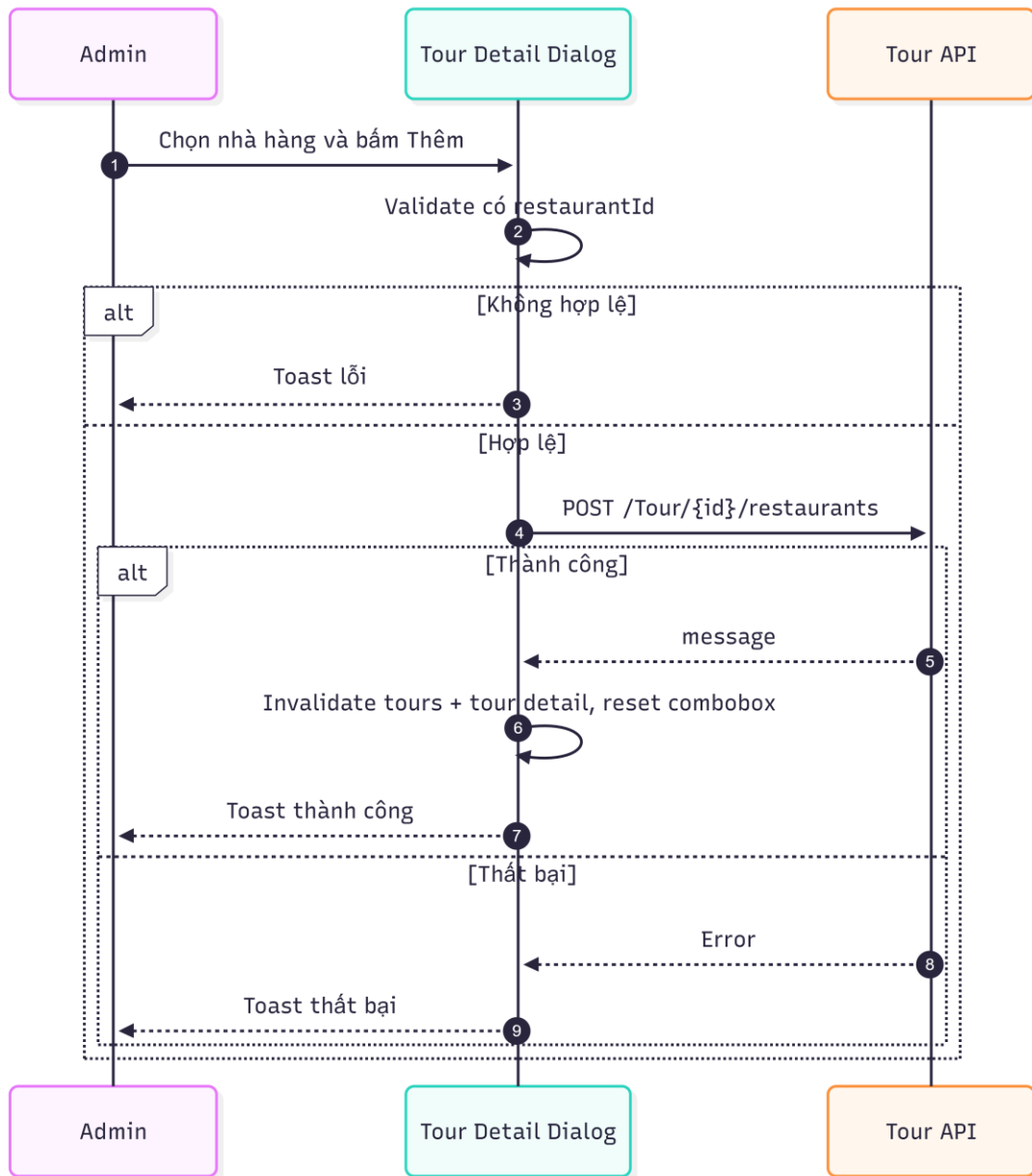
20_ThemNhaHangVaoTour.png
