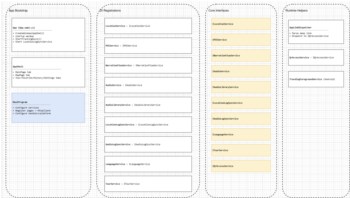
class_app.png
