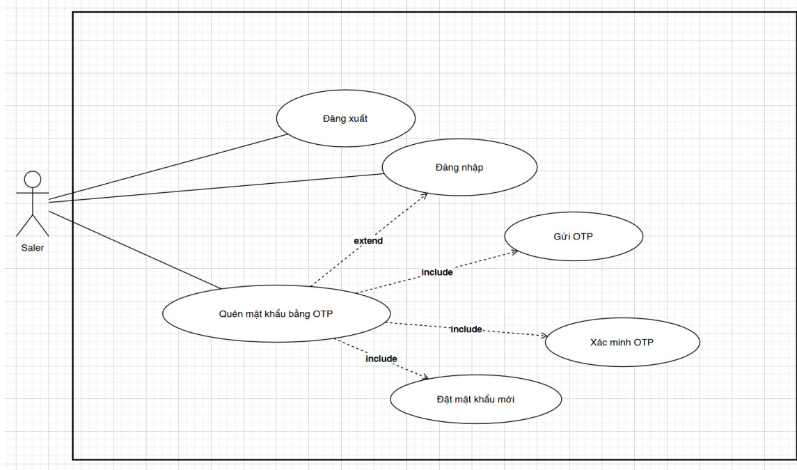
XacThuc.png
