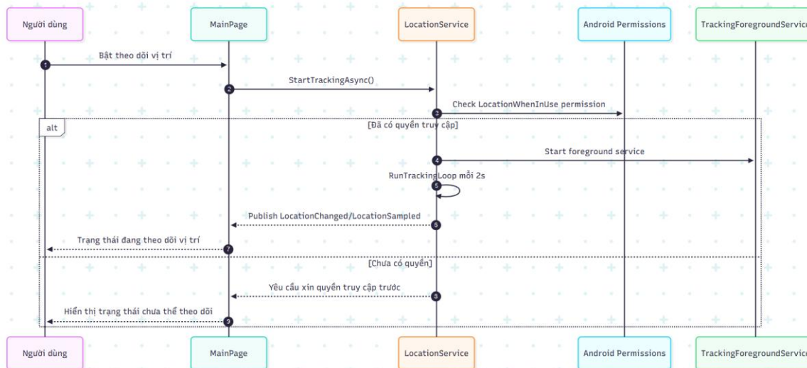
TheoDoiViTri.png
